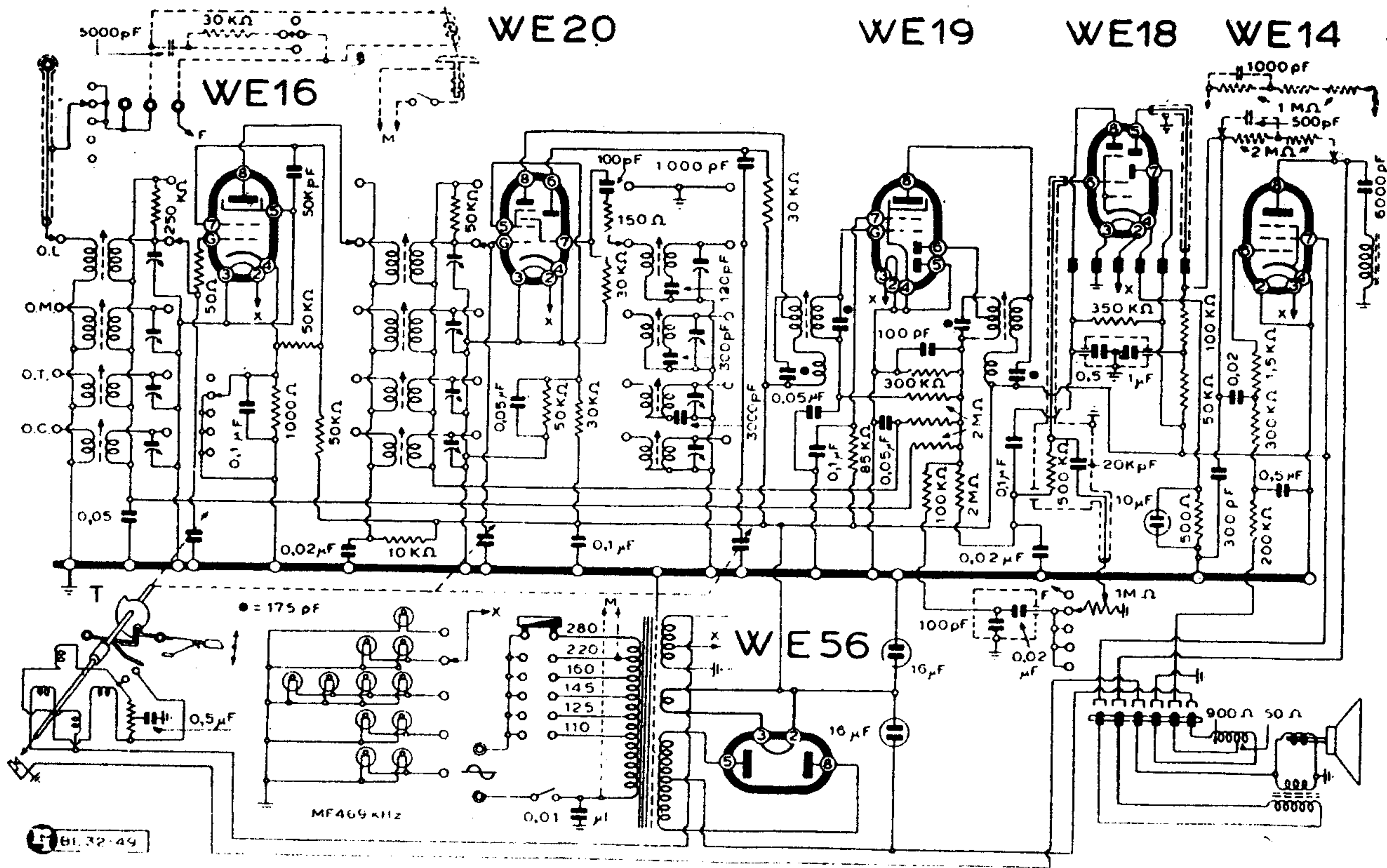
SIEMENS S. A. - MODD. « T 640 » « T 645 »
